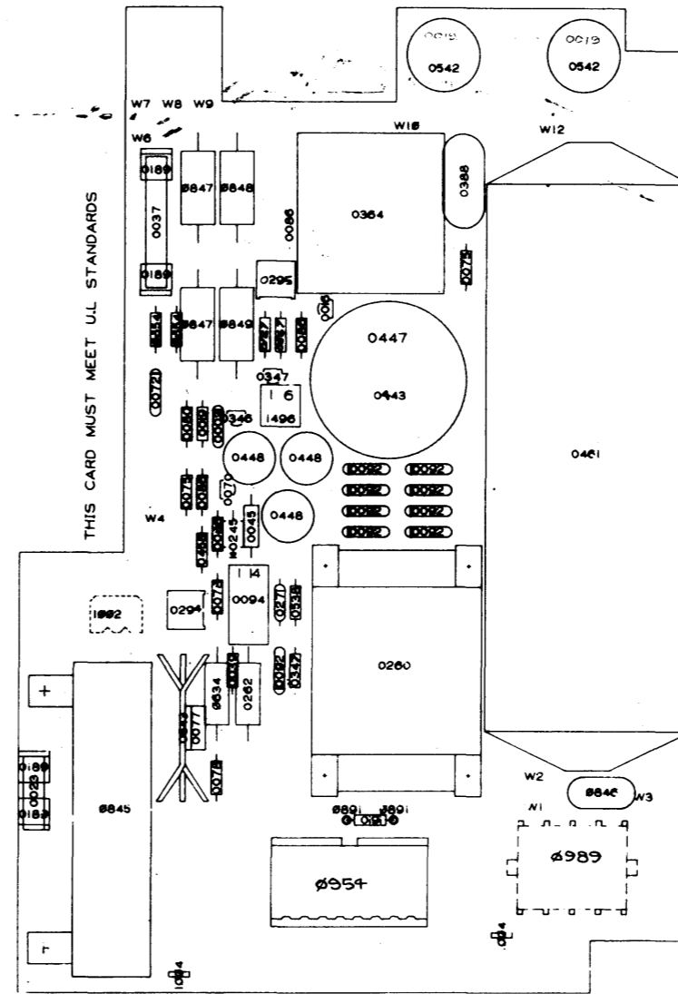
00300098505 LAYER 5
